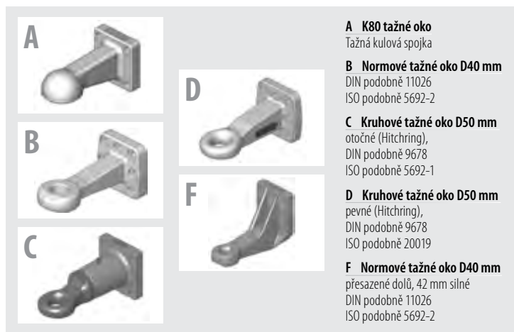
Tažná oka
